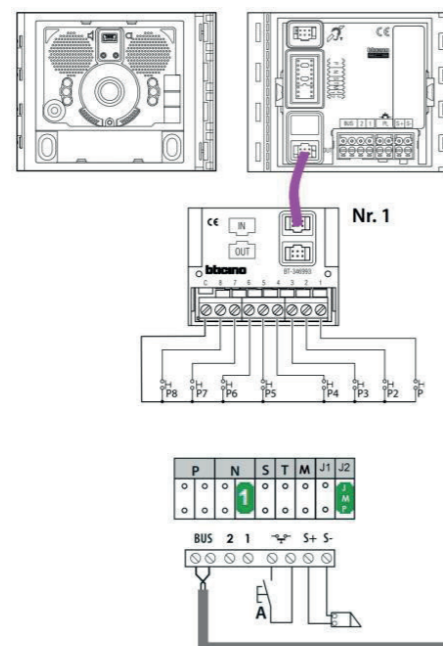
VOEDING Voorzien door elektricien Bticino Art 346050
