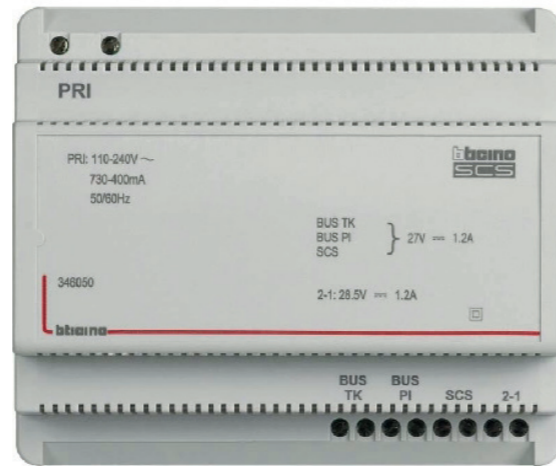
VOEDING Voorzien door elektricien Bticino Art 346050
